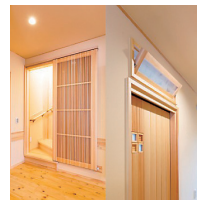
木製建具 赤松 / 桐
